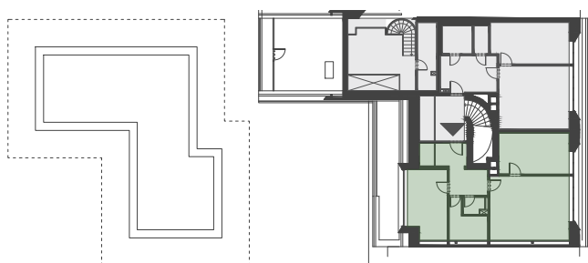
CELKOVÉ PŮDORYSNÉ SCHEMA PODKROVÍ
