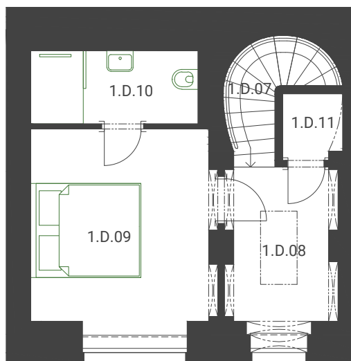
2.NP
