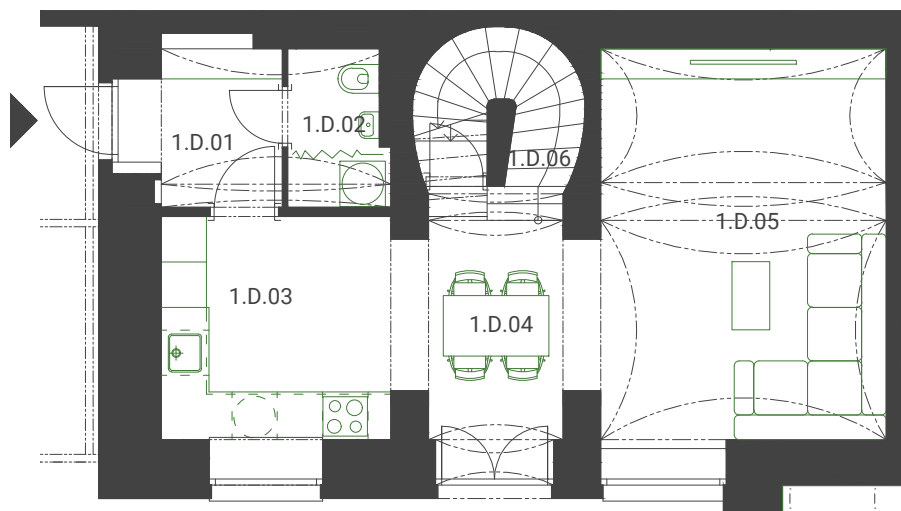
1.NP
