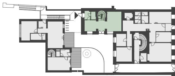
CELKOVÉ PŮDORYSNÉ SCHEMA 1.NP
